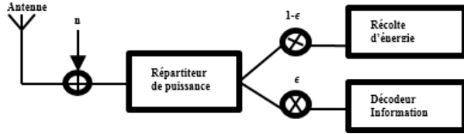
Figure 1.02 : Modèle de réseau Iot
