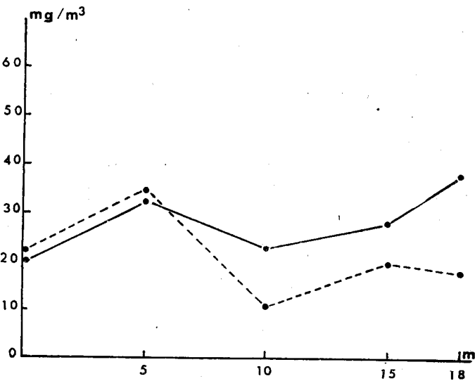
GRAPHIQUE N° 5. Pigments Station «V» — Chlorophylle C --- Caroténoïdes type Astacine ..... Caro. non Astacine
