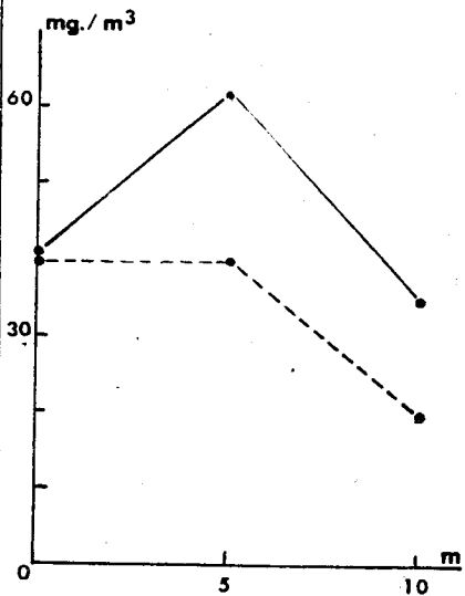
GRAPHIQUE N° 6 Station «L» Pigments — Chlorophylle A --- Chlorophylle B
