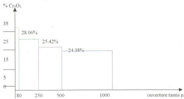
Fig 3 : Variation de teneur en Cr 2 O 3 (déchets de laverie)
